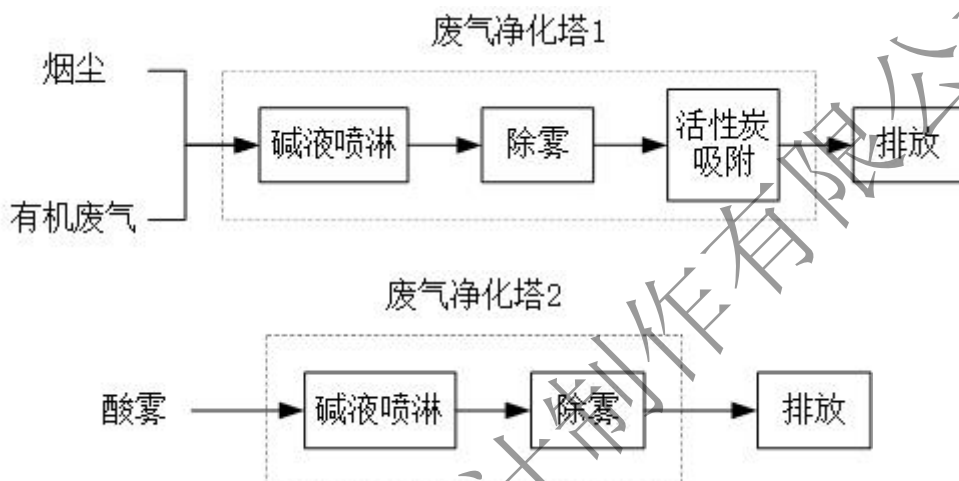
图 3 废气处理工艺流程图
