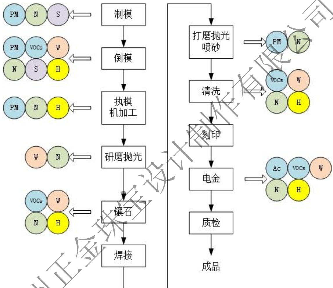
图 2 工艺流程和产污环节示意图
