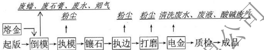
图 1 原有项目的生产工艺流程示意图（引自原有项目环评文件）
