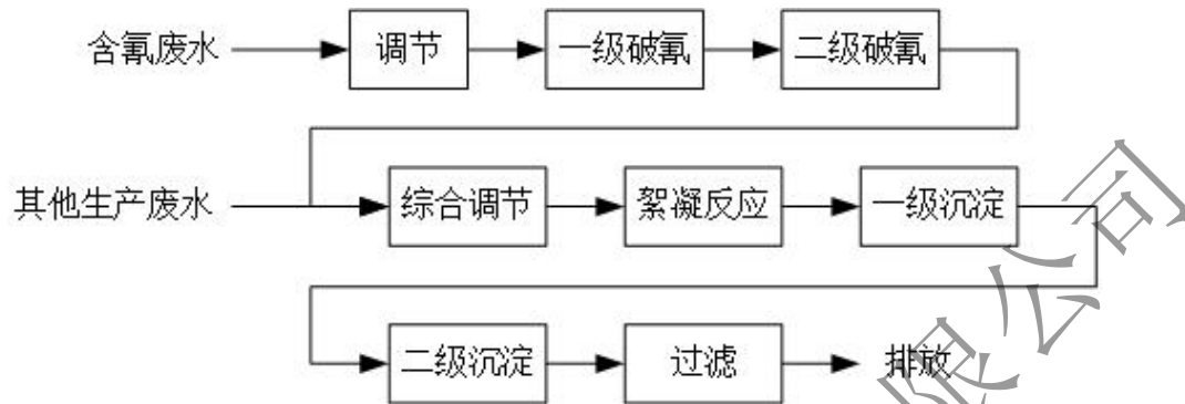
图 4 生产废水处理工艺流程图
